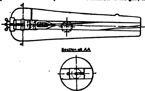
FIG. 9.—Wahrendorff Gun, 1846.
