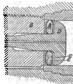
FIG. 52.—De Bange Obturator.
