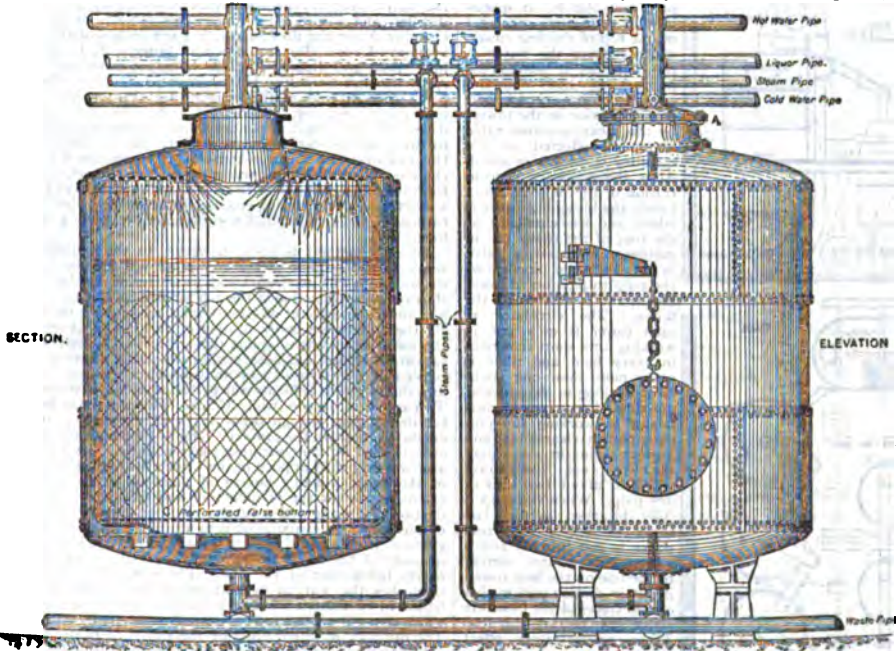
FIG. 3.—Sinclair Esparto Boiler.
