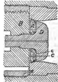
FIG. 53.—Steep Cone de Bange Obturator.
