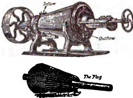
FIG. 9.—Jordan Beater.
