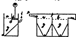
FIG. 7.—Harz Jig.
