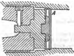
FIG. 47.—French Obturator.
