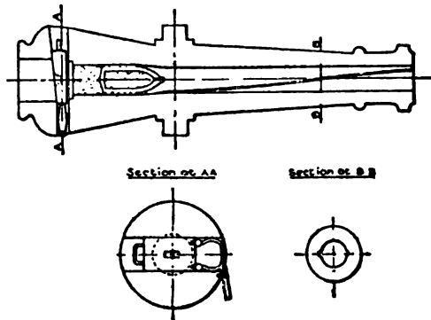
FIG. 8.—Cavalli Gun, 1845.
