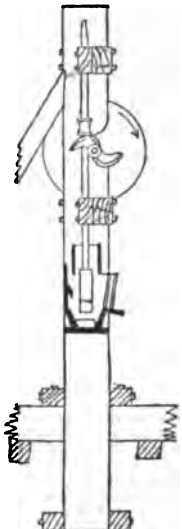
FIG. 4.—Gravity Stamp.
