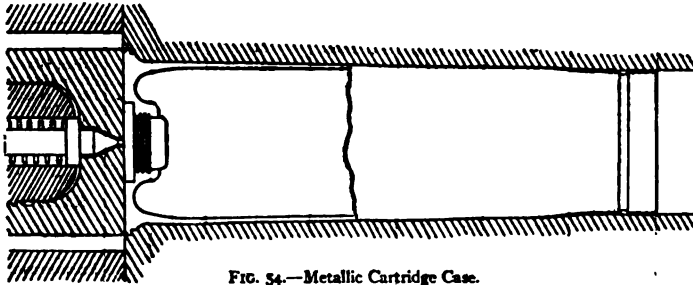
FIG. 54.—Metallic Cartridge Case.
