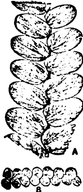
FIG. 5. A. Olosamites Beani . B. O. Bunburyanus . Inferior Oolite, England.
