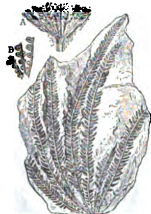
FIG. 8.— Matonidium Goepfertii . A. Summit of petiole. B. Fertile pinnules. Inferior Oolite, England.
